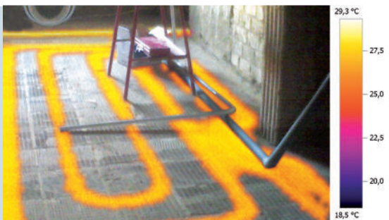
Verdeckte Rohrleitungen mit TwinPix auch im Echtbild erkennen
